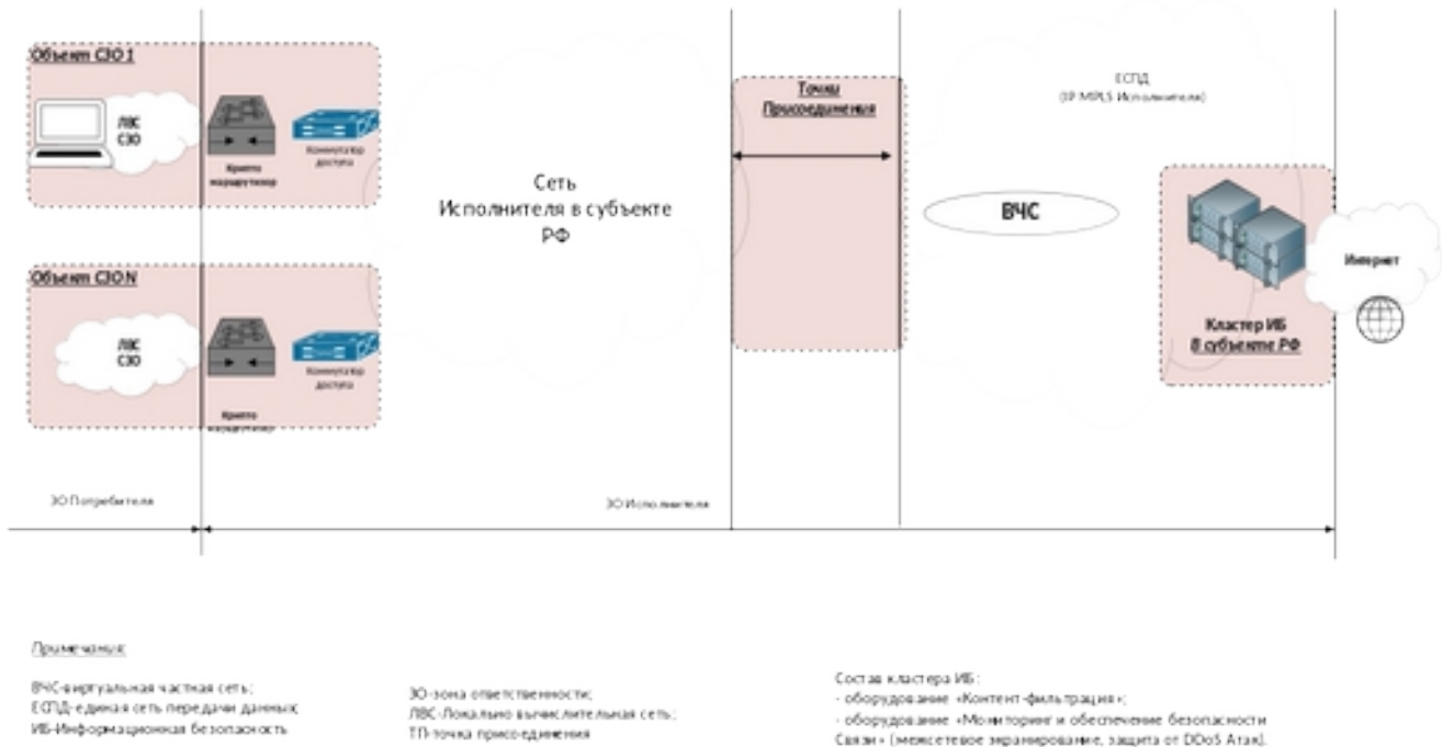
Рис. 5. Общая архитектура решений по контентной фильтрации.
