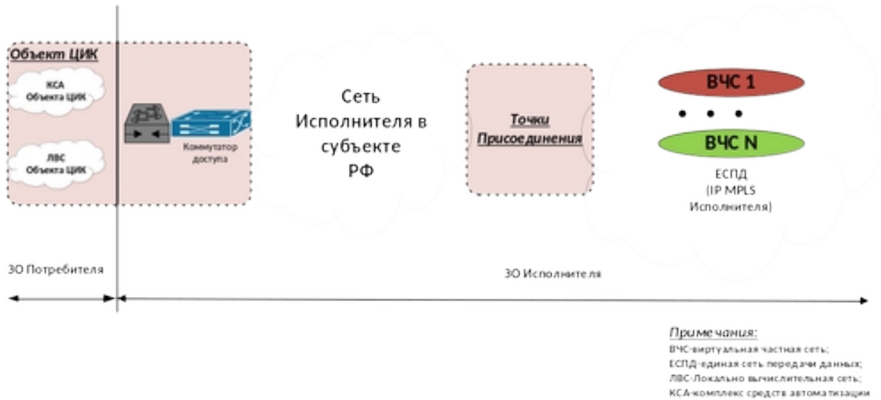
Рис.2. Архитектура Компонента «Предоставление доступа» для Объектов ЦИК.
